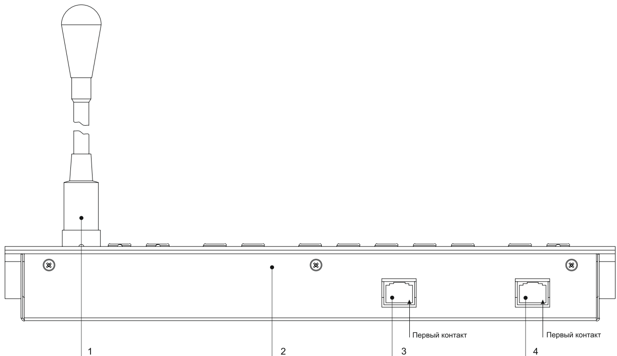
Рис. 2. Вид на Пульт со стороны разъемов.
