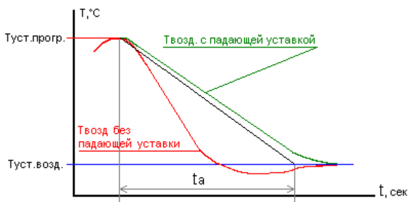
Рисунок 56. Падающая уставка
