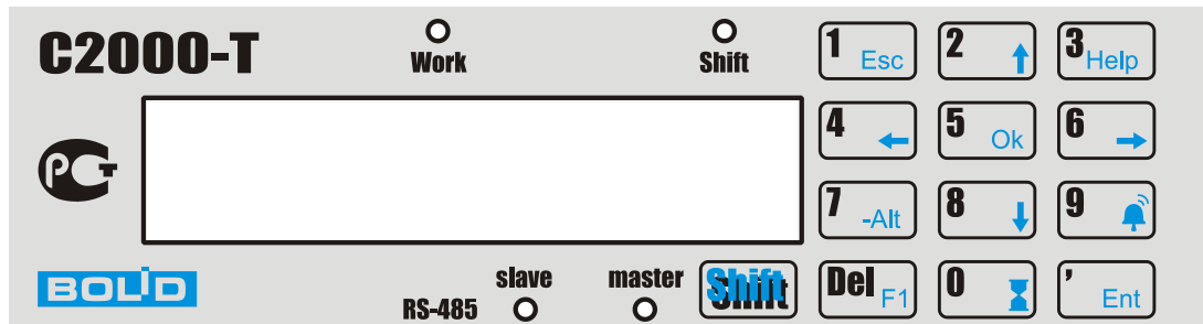
Рисунок 12. Элементы индикации и управления
